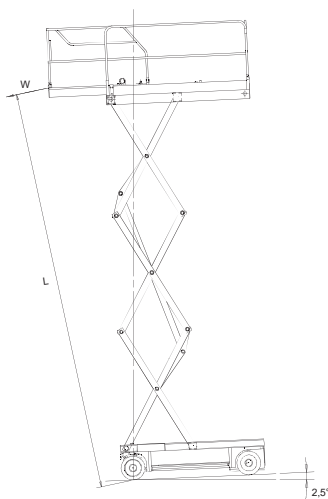
LONGITUDINAL POSITION
