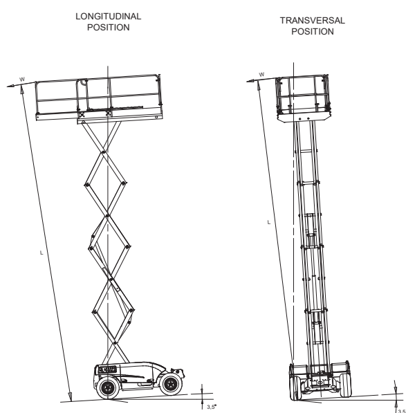
Estabilidade para COMPACT 12RTE (COMPACT 3368RTE)
