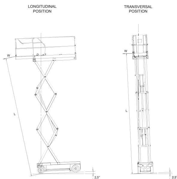
Estabilidade para C8W (COMPACT 2047E)
