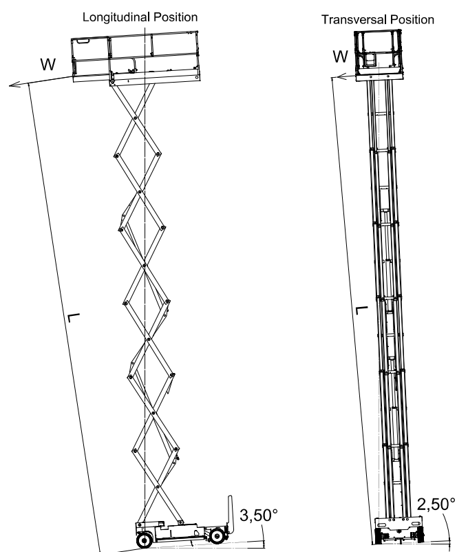
Estabilidade para COMPACT 14 (COMPACT 3947E)
