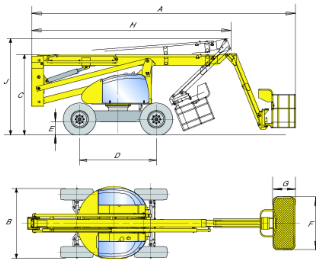
Esquema geral HA20PX - HA260PX
