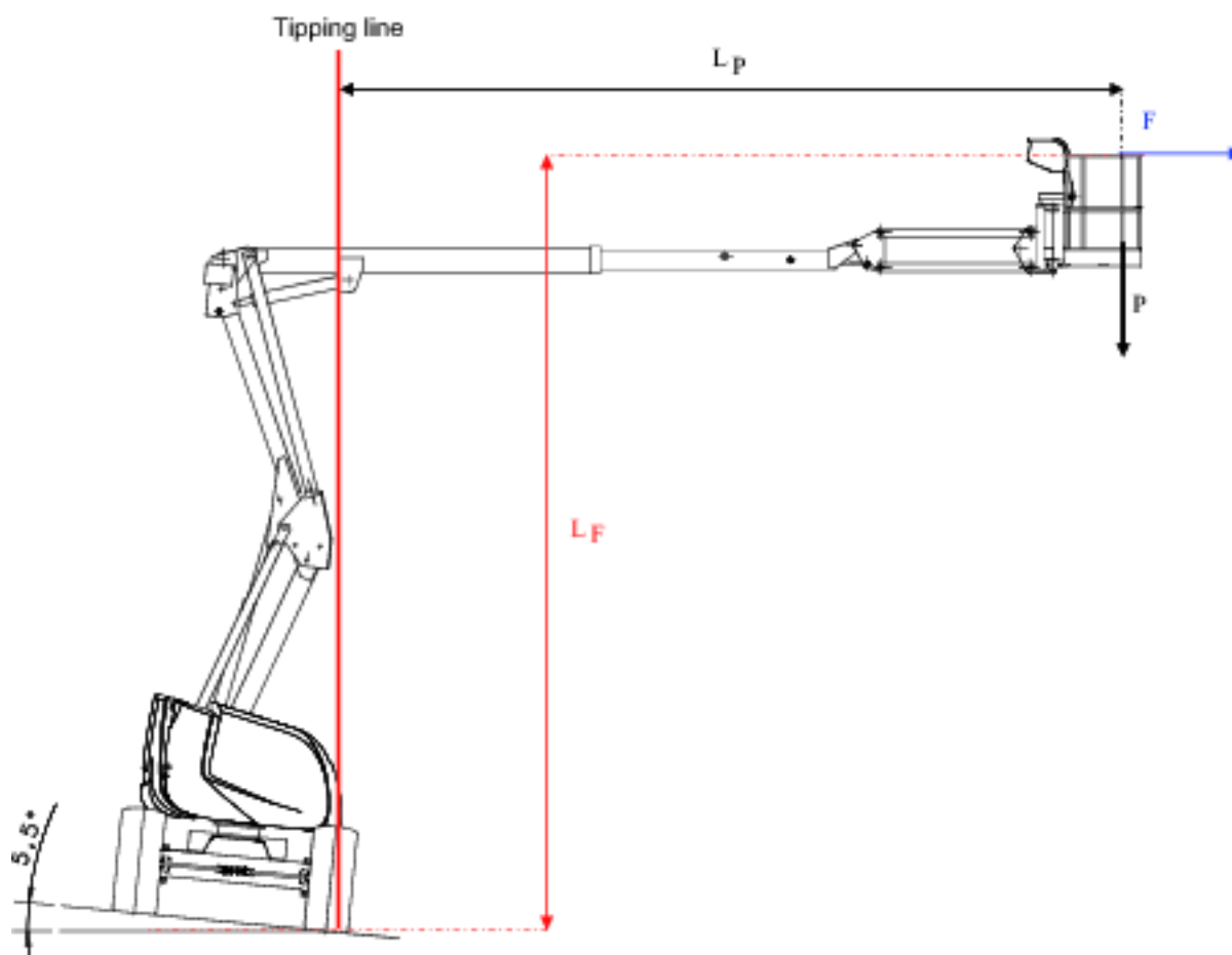
Quadro de estabilidade para HA120PX
